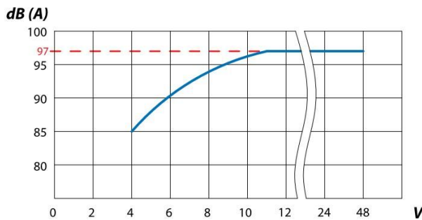
SAP-1302-C
