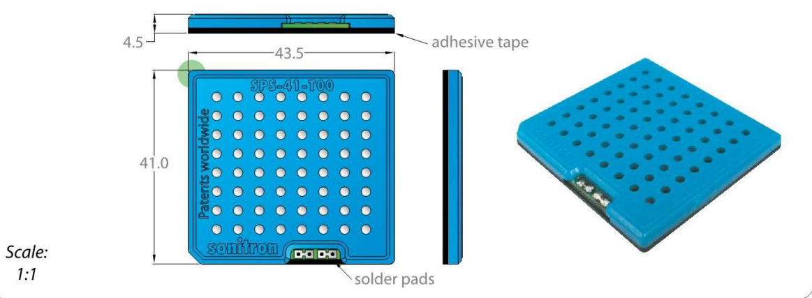
SPS-41-T00
