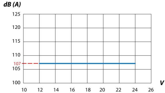
SAP-1302-B
