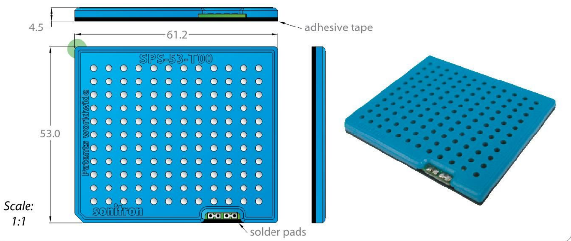
SPS-53-T00
