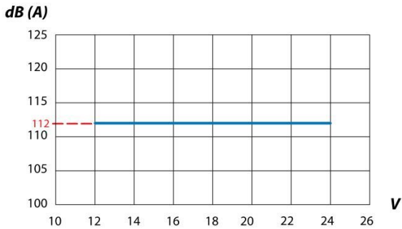
SAP-1302-A
